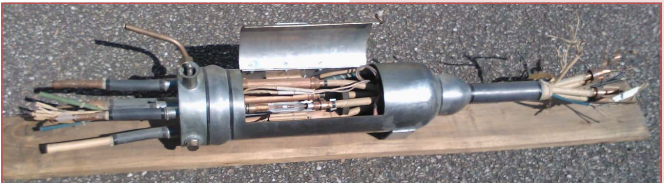
Câble ARRAS 175/01.
