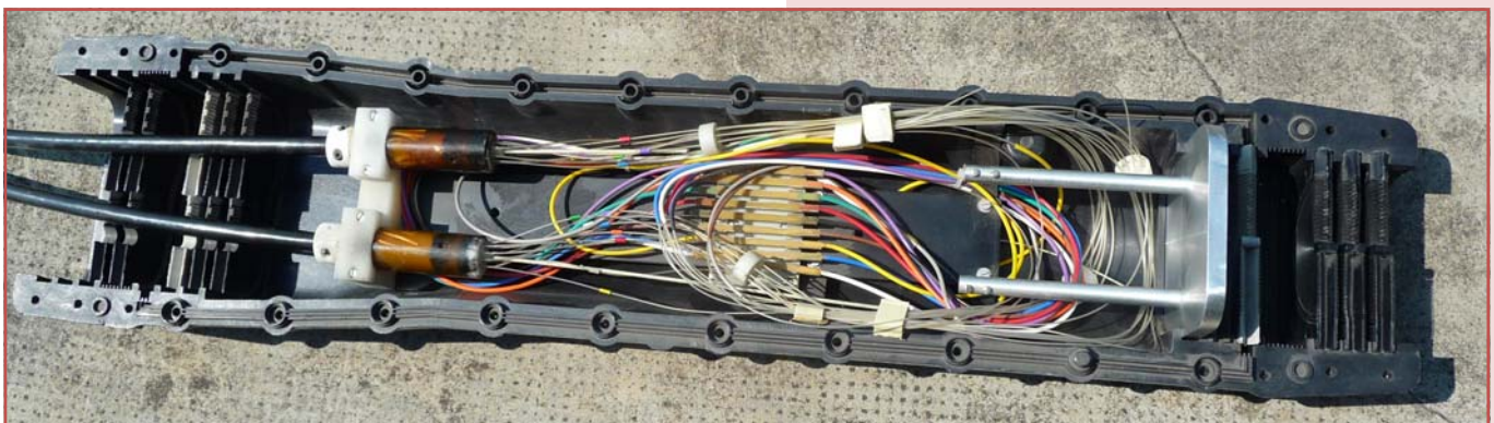
Raccord en fibres optiques.
